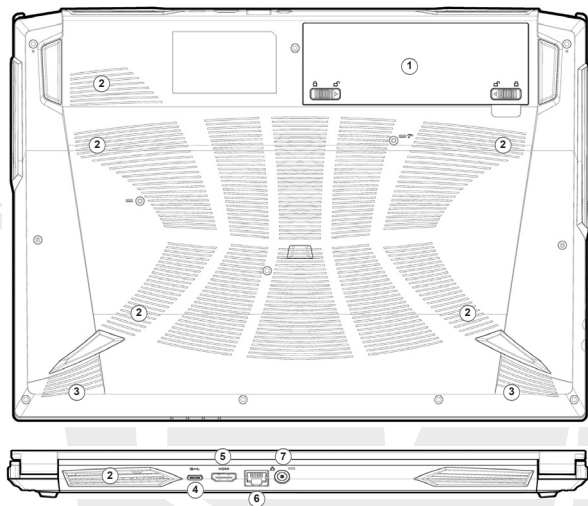
Abbildung 6 - Unter- und Rückansicht
