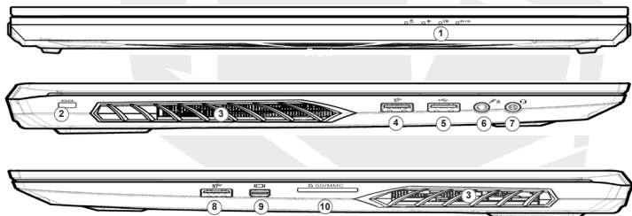
Figure 5 - Vues de l'avant, de la gauche et de la droite
