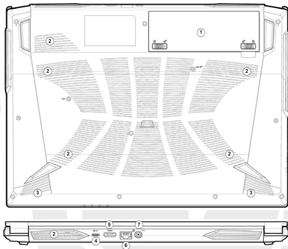
Figura 7 - Visualizzazione inferiore e posteriore
