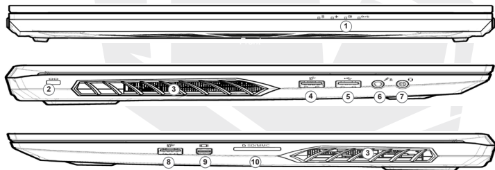
Figura 5 - Vistas frontal, izquierda y derecha
