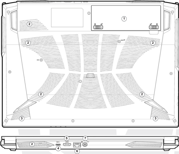
الشكل 7 الشكل من الأسفل والخلف
