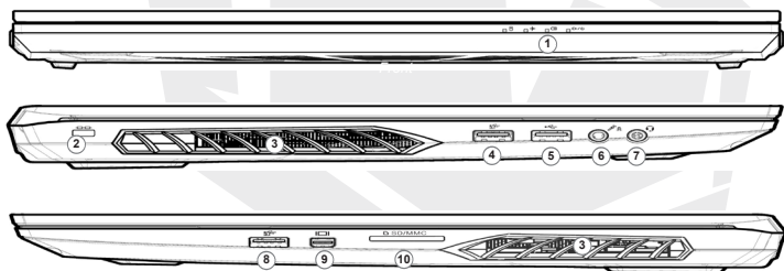
Figura 5 - Visualizzazioni anteriori, di sinistra e di destra
