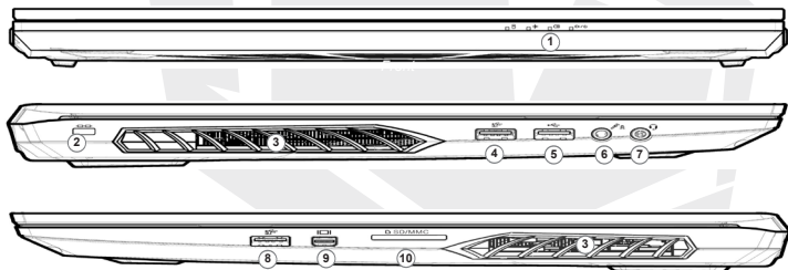
Abbildung 5 - Ansichten vorne, links und rechts
