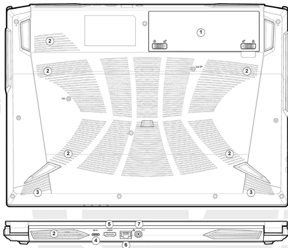
Figura 6 - Vistas inferior y posterior
