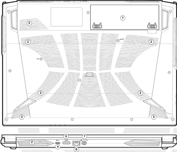
Şekil 6 - Alttan ve Arkadan Görünümler
